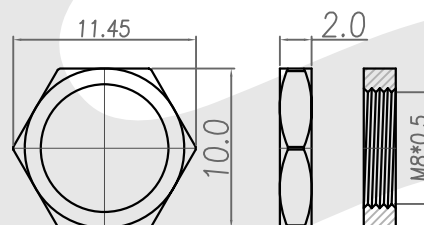
NUT
